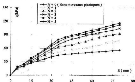
Figure 8 : Influence du nombre de nappes de morceaux plastiques (pour : H/B=0.2 ; \Delta y=4 \text{ cm} ; S=6 \times 30 \text{ cm}^2 ; M=150 \text{ g}=1.66 \text{ Kg/m}^2 )
