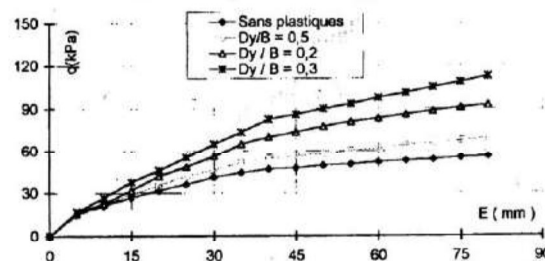
Figure 10 : Influence de l'espacement des nappes des morceaux plastiques (pour : N=4 ; H/B=0.2 ; S=30 \times 6 \text{ cm}^2 ; M=150 \text{ g}=1.66 \text{ Kg/m}^2 )
