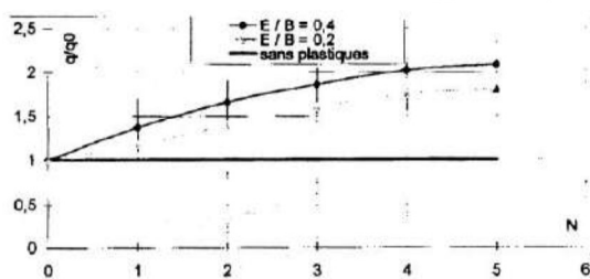
Figure 9 : Evolution de R.C.P. en fonction du nombre de nappes de matières plastiques (pour : H/B=0.2 ; \Delta y=4 \text{ cm} ; S=6 \times 30 \text{ cm}^2 ; M=150 \text{ g}=1.66 \text{ Kg/m}^2 )
