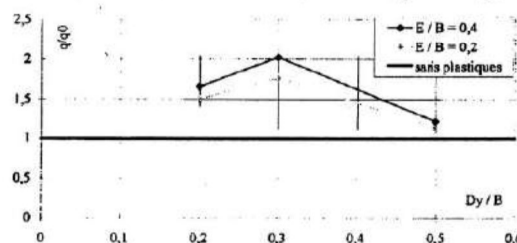
Figure 11 : Variation de R.C.P. en fonction de l'espacement des nappes de morceaux plastiques (pour : N=4 ; H/B=0.2 ; S=30 \times 6 \text{ cm}^2 ; M=150 \text{ g}=1.66 \text{ Kg/m}^2 ).
